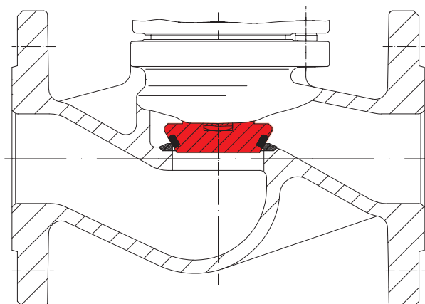
锥形阀头，阀头与阀座带司太尔合金
