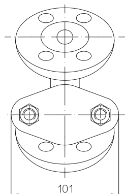
仅限于DN15: 滤网底盖视图（不锈钢除外）
